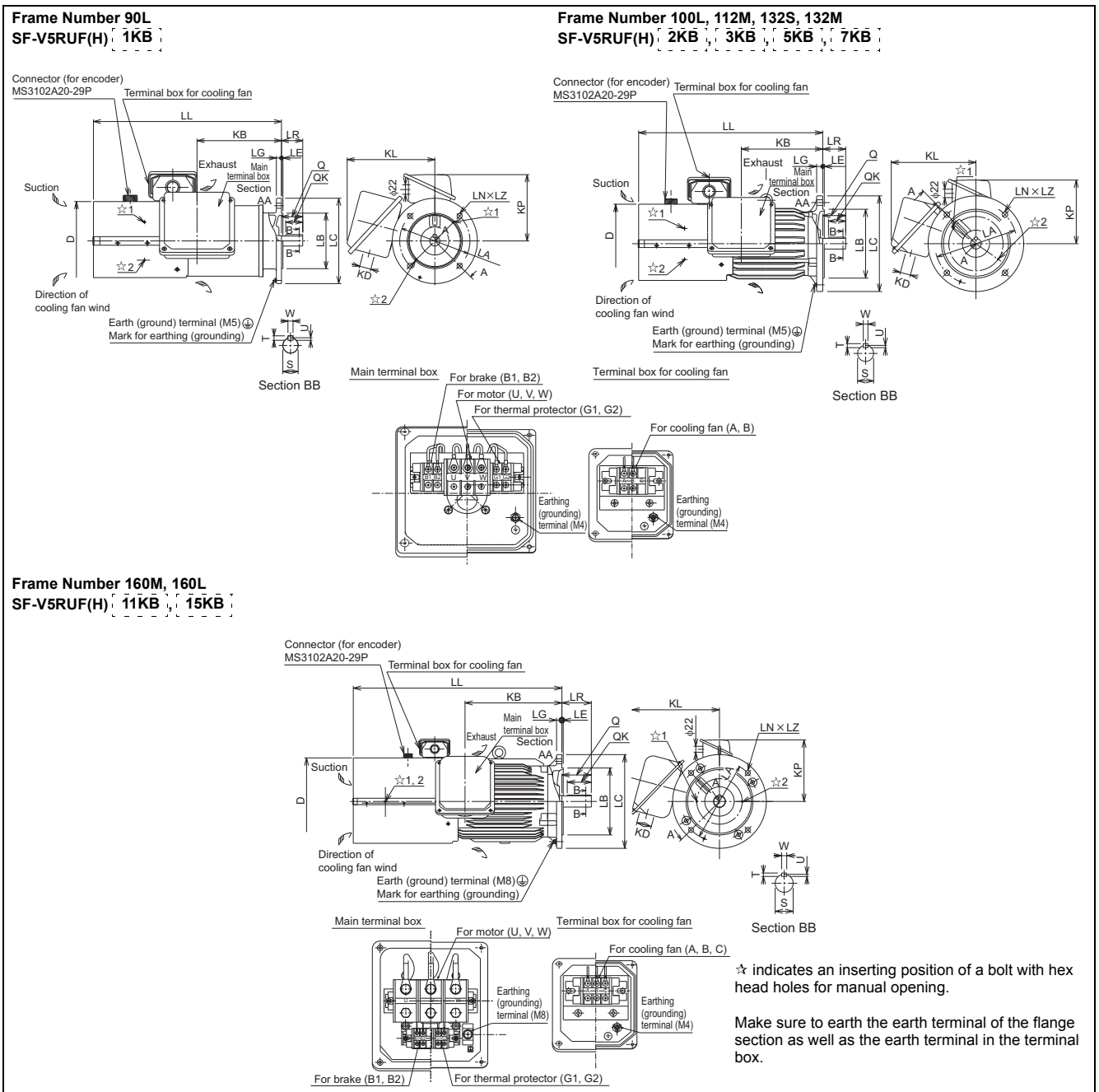
Dimensions table
