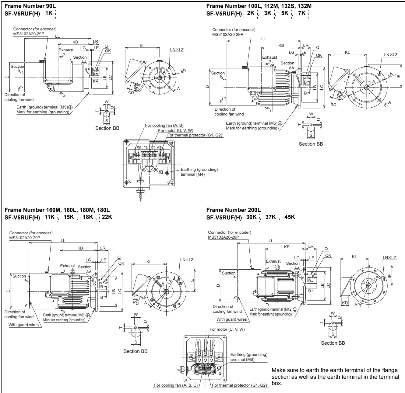
Dimensions table
